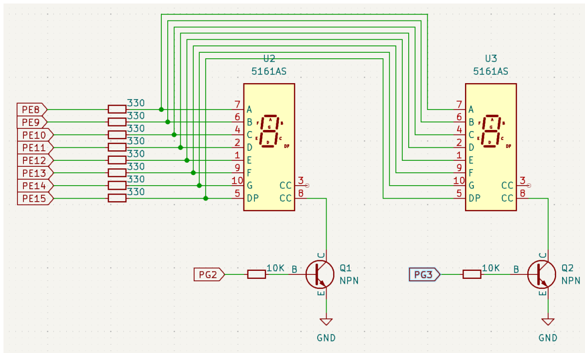
Hình 2: Ghép nối 2 module LED 7 thanh
