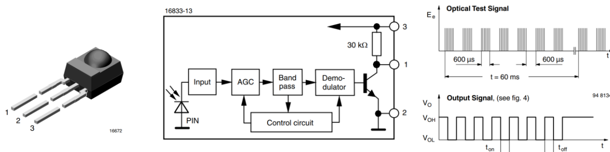
Hình 3: Nguyên tắc hoạt động của bộ thu HS0038
